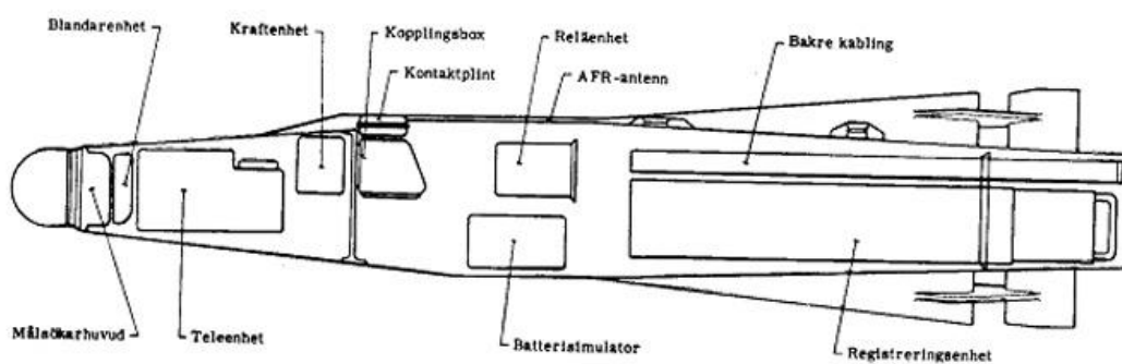
ÖVNINGSROBOT 27
