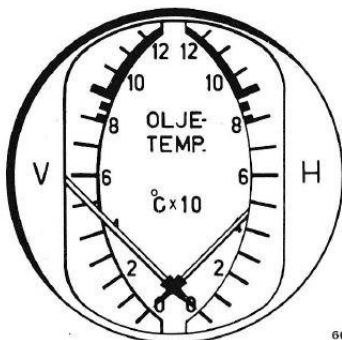
Bild 43. Oljetermometer (4:43)
