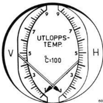
Bild 41. Utloppstermometer (4:33)
